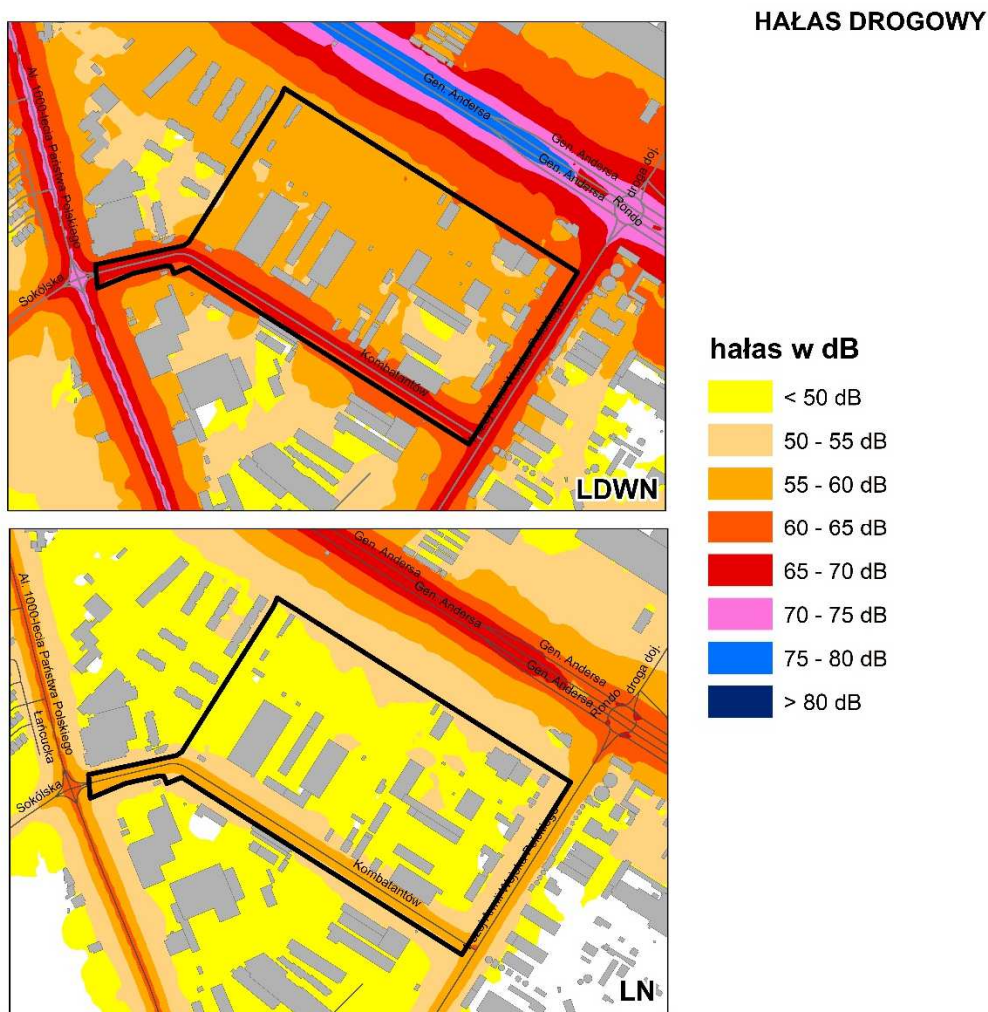
Rysunek 5 Imisja hałasu komunikacyjnego L_{DWN} i L_N w obszarze objętym projektem planu źródło: Strategiczna mapa hałasu miasta Białystok, 2022 r.
