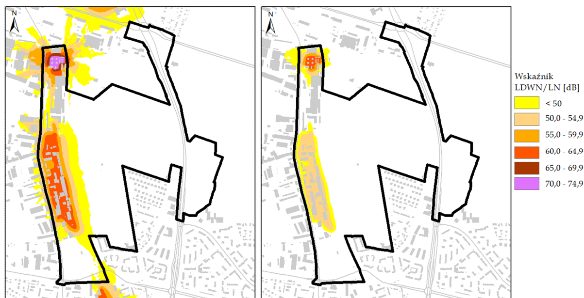
Rysunek 18 Imisja hałasu przemysłowego LDWN i LN w obszarze objętym projektem planu
