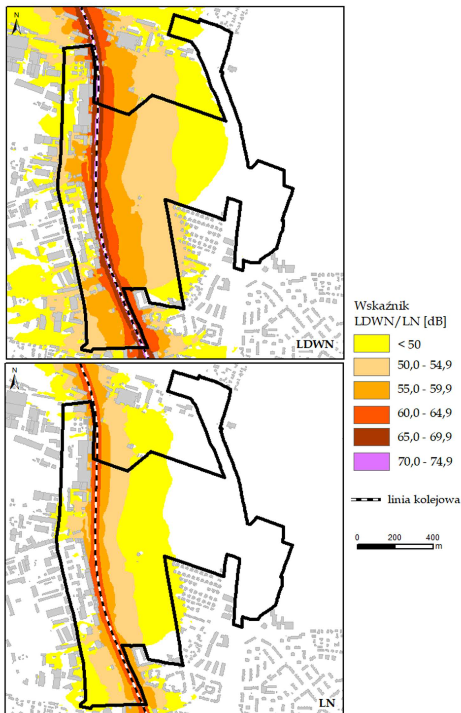
Rysunek 17 Imisja hałasu kolejowego L_{DWN} i L_N w obszarze objętym projektem planu źródło: Strategiczna mapa hałasu miasta Białystok, 2022 r.
