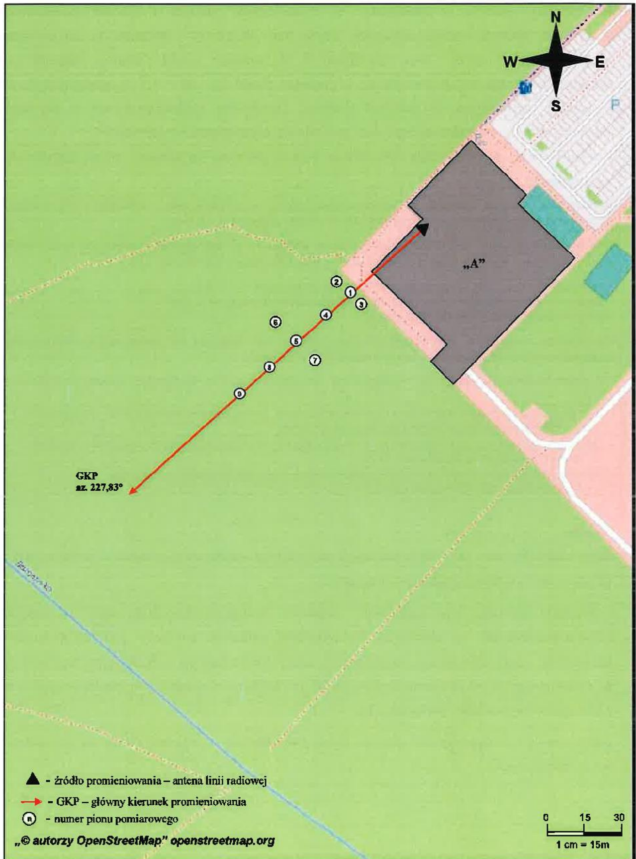
Rys. 1. Usytuowanie punktów i pionów pomiarowych w otoczeniu instalacji radiokomunikacyjnej Stacja Netia BIALB185-BIALM00112 Białystok, Aleja Jana Pawła II 51
