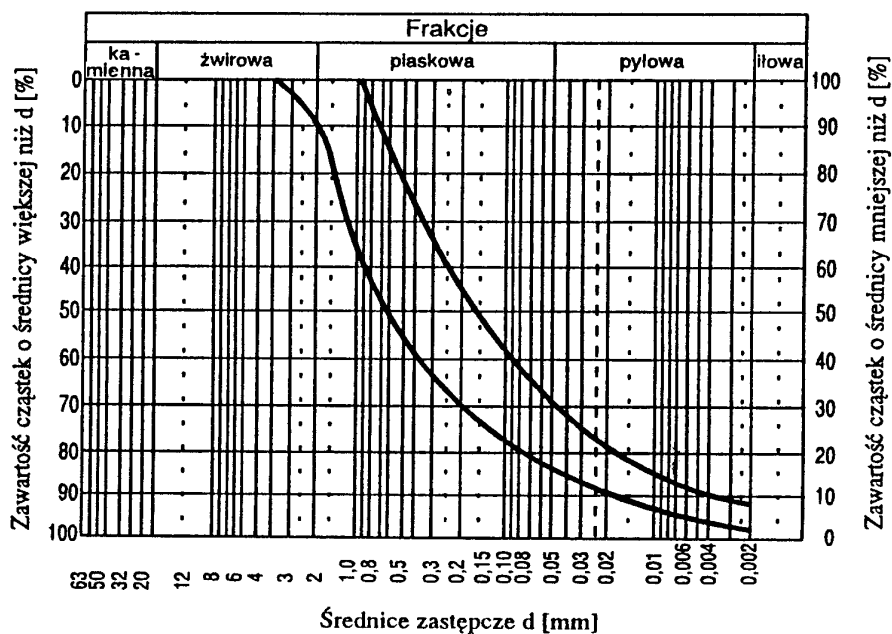
Tablica 2. Ramowy skład uziarnienia optymalnej mieszanki gliniasto-żwirowej
