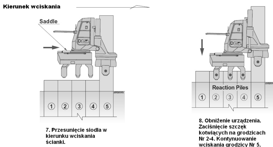
Rysunek 1. Procedura wciskania grodzic urządzeniem samokroczącym
