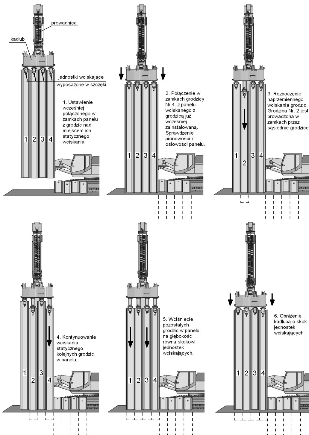
Rysunek 2. Procedura wcisnięcia grodzic urządzeniem mocowanym do masztu prowadzącego
