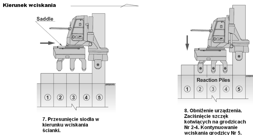
Rysunek 1. Procedura wciskania grodzic urządzeniem samokroczącym
