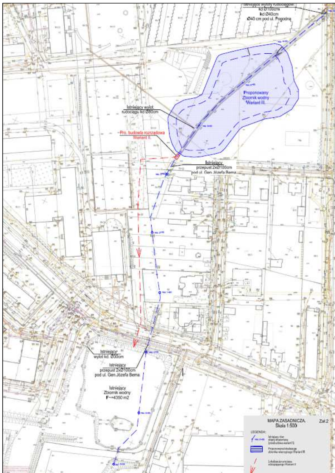
Rycina 7 Wariant II i III rozwiązania problemu funkcjonowania (przepustowości) rowu
