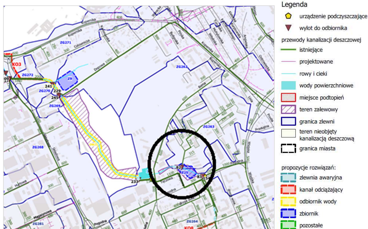
Rycina 8 Analiza hydrauliczna istniejącego systemu kanalizacji deszczowej miasta Białegostoku.
